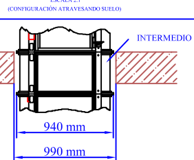
DETALLE "A" ESCALA 2:1
